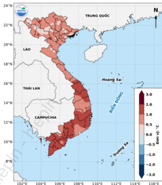
Hình 2. Phân bố chuẩn sai nhiệt độ trung bình mùa 3 tháng 6-8 năm 2026 (°C)
