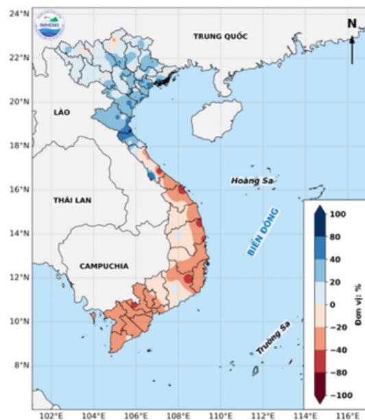
Hình 4. Phân bố chuẩn sai lượng mưa mùa 3 tháng 6-8 năm 2026 (%)
