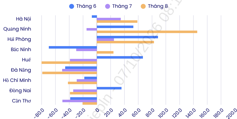
Hình 3. Chuẩn sai lượng mưa trung bình tháng (6-8/2026) tại các thành phố trực thuộc Trung ương (đơn vị: %)
