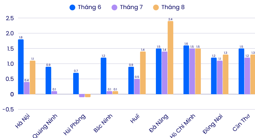
Hình 1. Chuẩn sai nhiệt độ trung bình tháng (6-8/2026) tại các thành phố trực thuộc Trung ương (đơn vị: °C)
